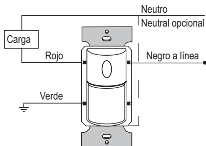
Cableado de nivel simple
