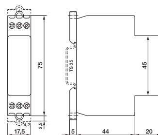
Dimensions
