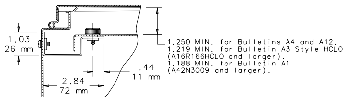
DETAIL Y
